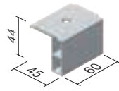
端部パネル押え (パネル厚40mm用) 品番:TYKEA-40-M
