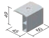
端部パネル押え (パネル厚45mm用) 品番:TYKEA-45-M
